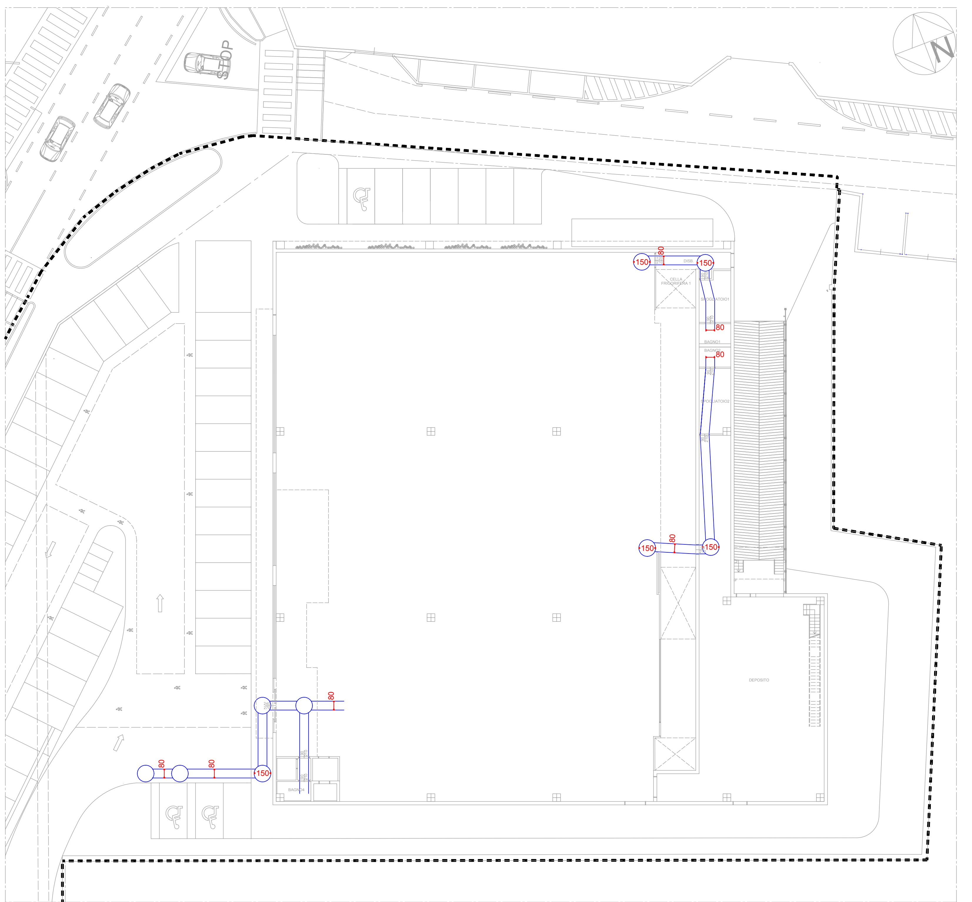
VERIFICA ACCESSIBILITA' E VISITABILITA' I. 13/89 scala 1:200
