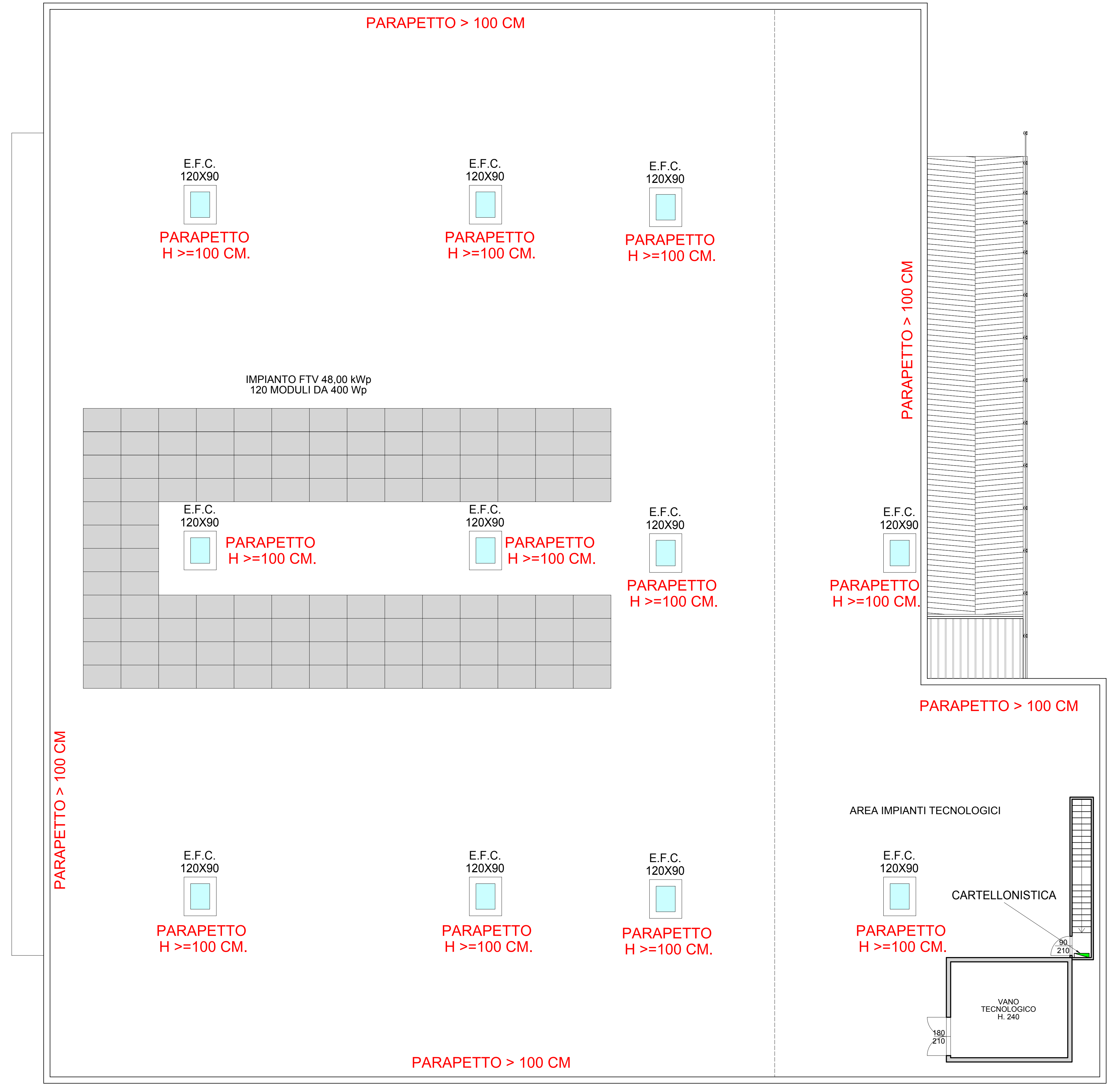
PIANTA INDIVIDUAZIONE DISPOSITIVI CONTRO LE CADUTE DALL'ALTO scala 1:100
