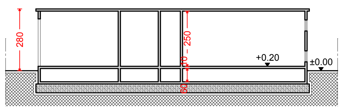
SEZIONE AA scala 1:100
